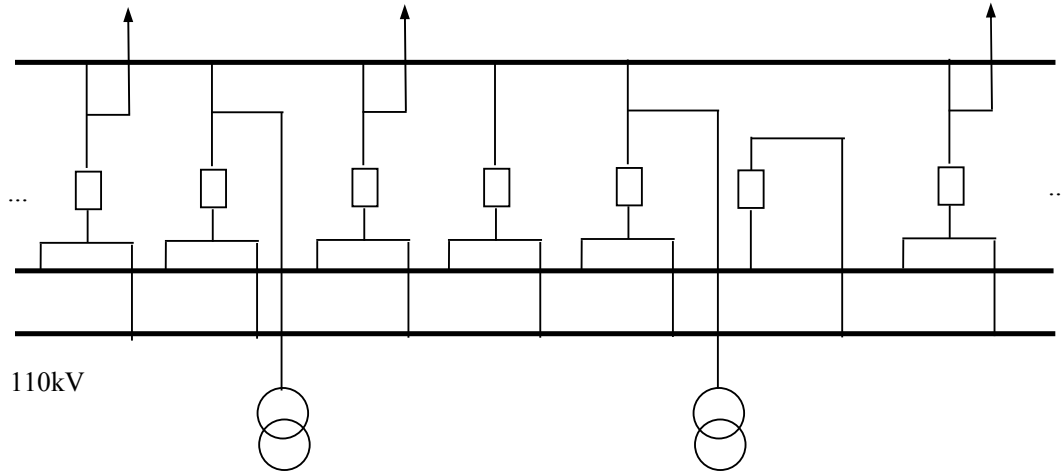
Hình 1. Sơ đồ 02 thanh cái và thanh cái vòng – MC vòng và MC liên lạc riêng
