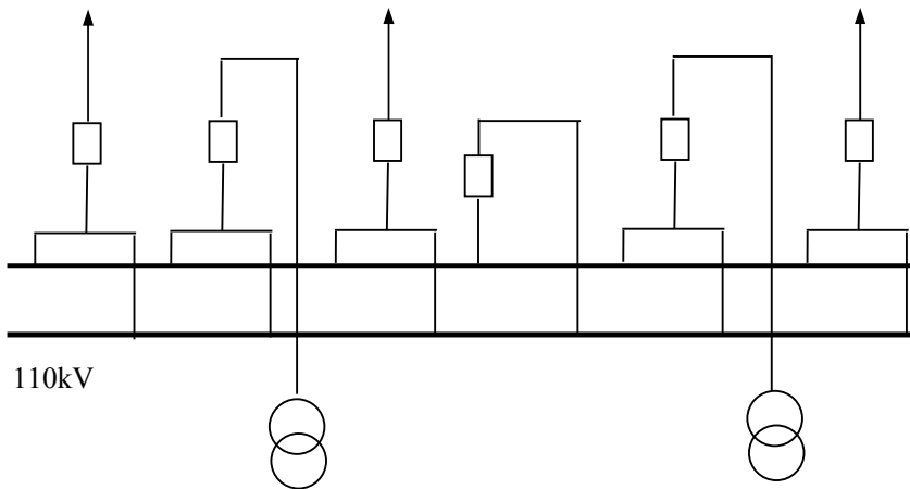
Hình 2. Sơ đồ 02 thanh cái chính có MC liên lạc
