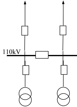
Hình 4. Sơ đồ chữ H
