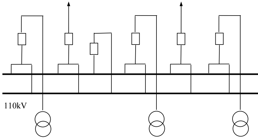
Hình 2a. Sơ đồ 02 thanh cái chính có MC liên lạc và 03 MBA
